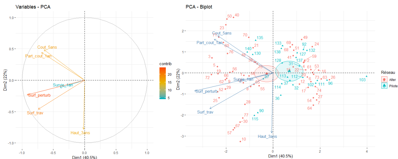
Figure A2.1 : à gauche représentation des variables sur les deux premiers axes de l'ACP sur le maximum d'individus et 6 variables ; à droite, représentation des différents placeaux colorés par réseau, avec les valeurs moyennes et ellipses de confiance à 95% de ces valeurs.
