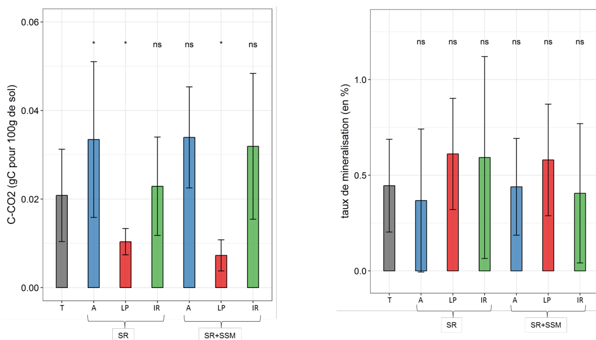
Figure A1.4 : Minéralisation potentielle du COS dans l'horizon 0-10 cm à l'échelle du transect (A = andain ; LP = ligne de plantation ; IR = inter-rang) pour les 3 modalités. A / Minéralisation potentielle du C exprimée en C dégagé sous forme de CO 2 sur les 7 jours d'incubation (gC-CO 2 .100g -1 de sol) ; B/ Taux de minéralisation du C (% du COT). (* = significatif à p < 0,05 ; ns = non significatif ; Kruskal-Wallis).
