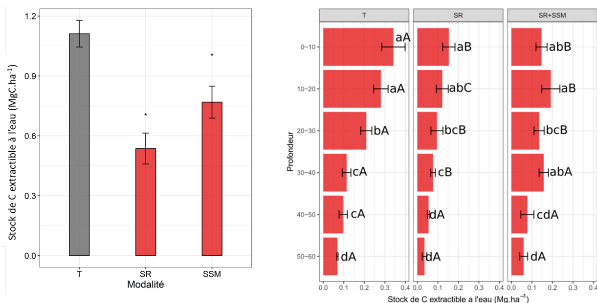
Figure A1.6 : Stocks de C organique extractible à l'eau sur 0-60 cm (en \text{MgC.ha}^{-1} ) et répartition de ces stocks de C dans le profil de sol de la ligne de plantation pour les 3 modalités à Bord-Louviers. Des minuscules différentes indiquent les différences au sein du profil de sol par modalité, des majuscules différentes indiquent les différences entre modalité (Kruskal-Wallis, p < 0,05 ).
