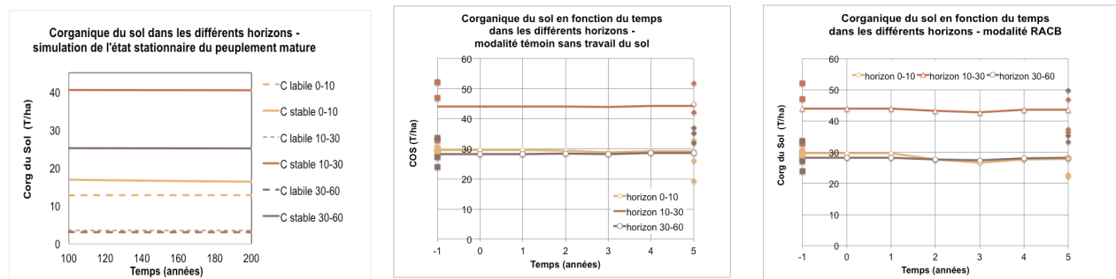
Figure A3. 4: simulations réalisées par le modèle. a- état stationnaire du peuplement mature réalisé sur un siècle. b- peuplement témoin, c peuplement avec travail du sol par RACB. La coupe a lieu juste après le temps 0. On considère qu'il n'y a pas d'apports de rémanents de coupe, on néglige également les apports des souches et du système racinaire. Les points correspondent aux données observées, les courbes aux données simulées.
