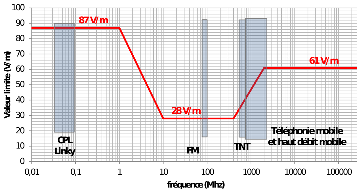
Figure 2 : Valeurs-limites fixées par le décret du 3 mai 2002 en champ électrique exprimé en V/m
