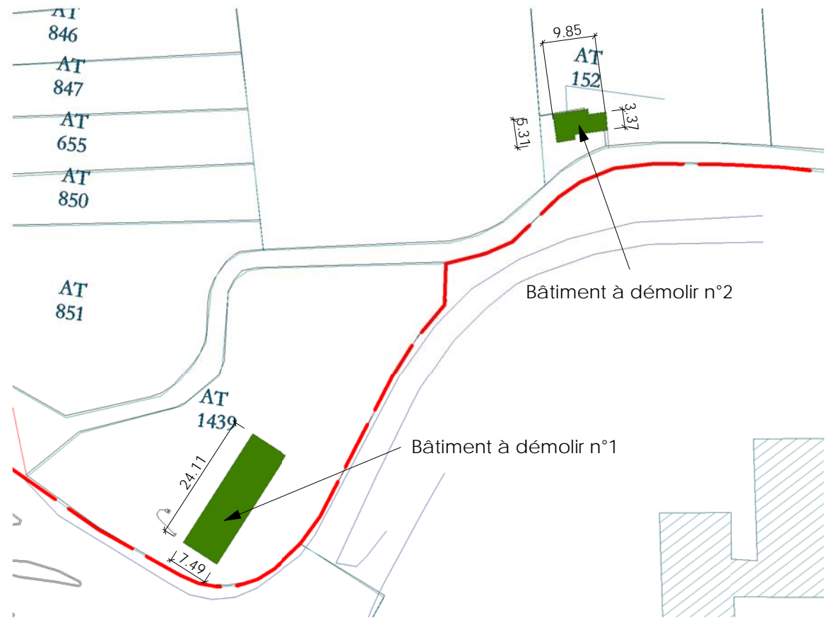
2 DETAIL BÂTIMENTS A DEMOLIR Ech : 1 : 1000
