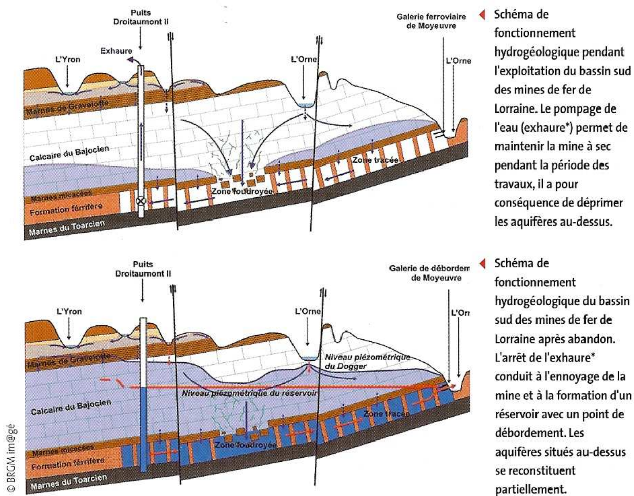
Figure 11 : Schéma de fonctionnement hydrogéologique du bassin ferrifère sud lorrain, avant et après arrêt de l'exhaure (source : BRGM)
