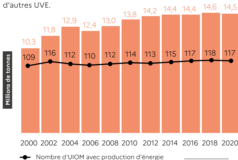
Figure 33 Évolution des tonnages incinérés avec production d'énergie
