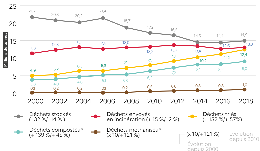
Figure 15 Évolution des tonnages traités dans les installations de traitement des déchets municipaux
