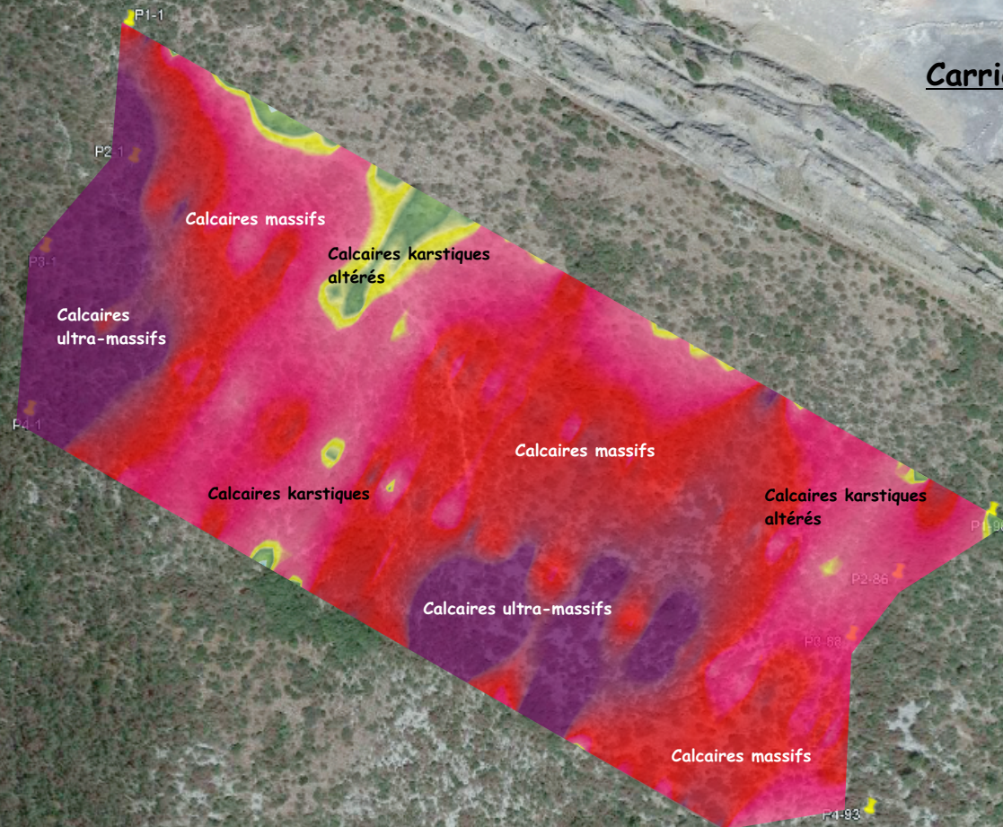
Carte 1: Carte des résistivités à la profondeur de 2.0 mètres
